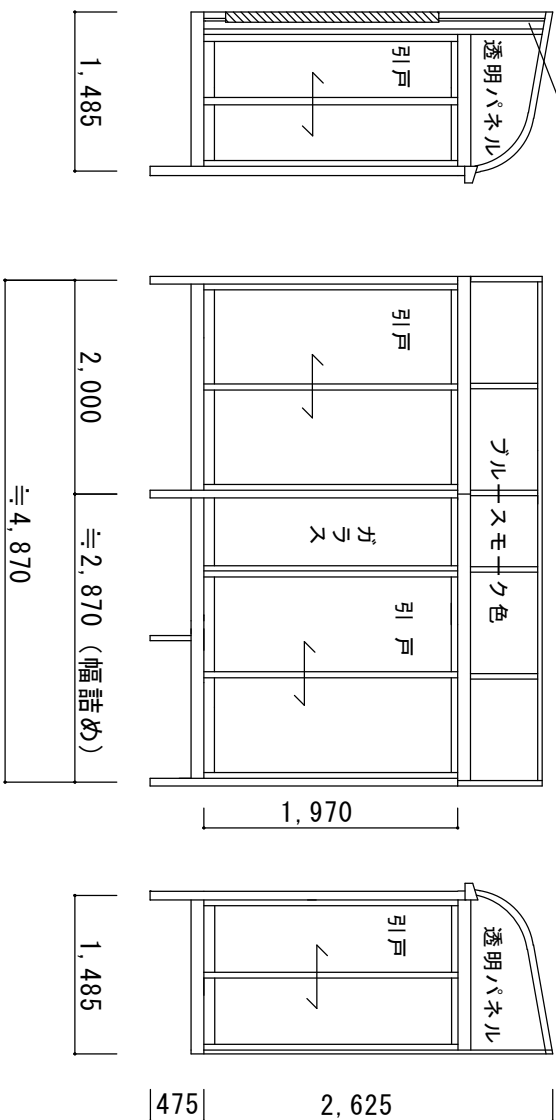
立面図 戸袋逃げパネルは透明となります。
