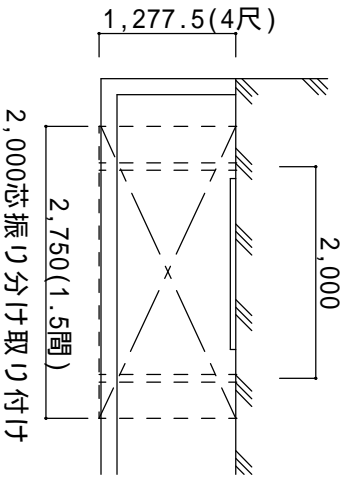
平面図
