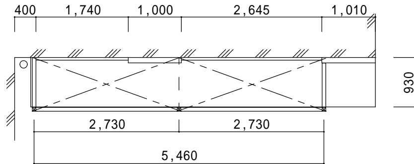
平面図
