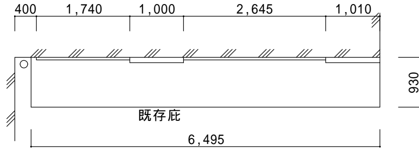
現状図
