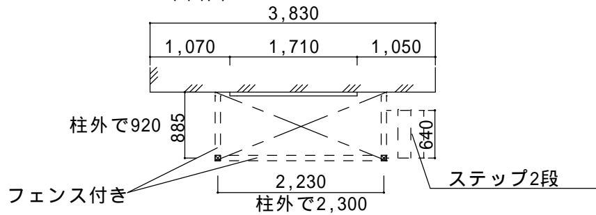
平面図
