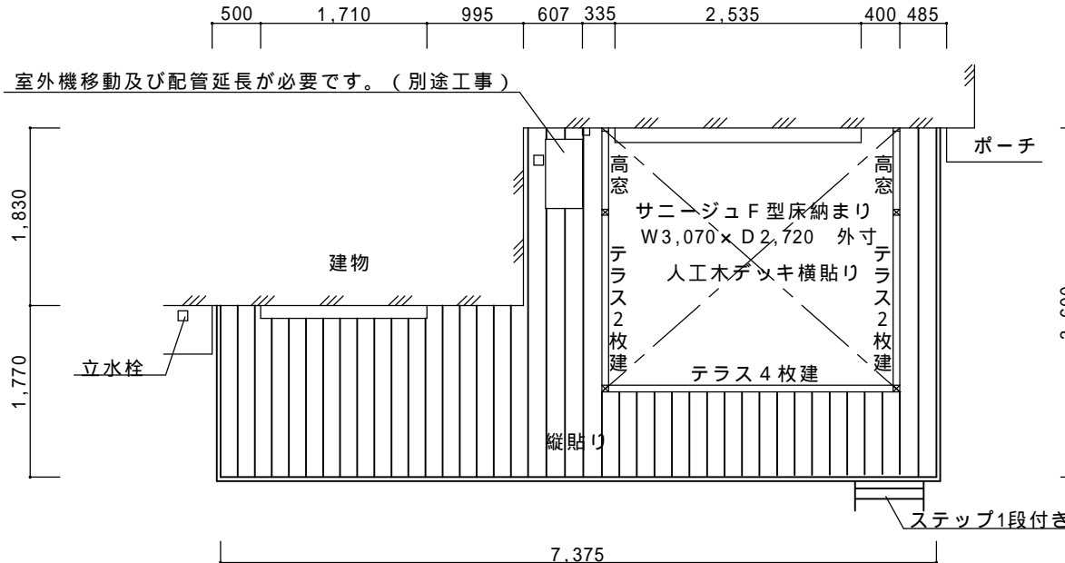
サニージュF型床納まり+樹ら楽ステージ平面図
