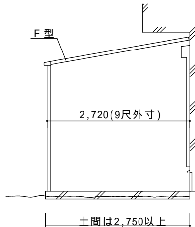
プラン F型 間口1.0間×出幅9尺 側面図
