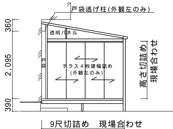
プラン 出幅9尺側面図
