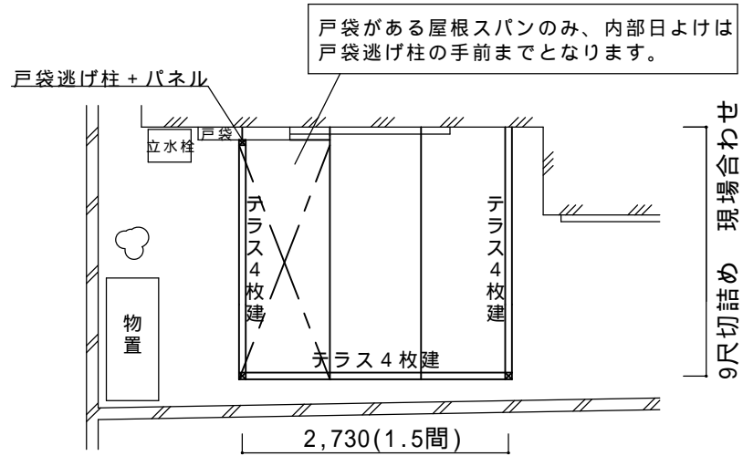
プラン 出幅9尺平面図
