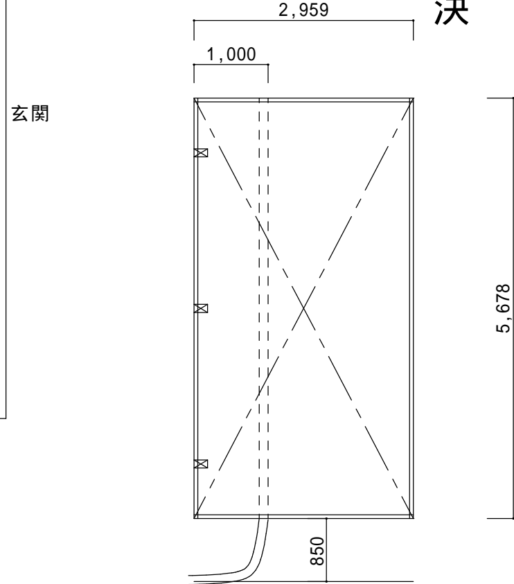
ファインポート Z平面図
