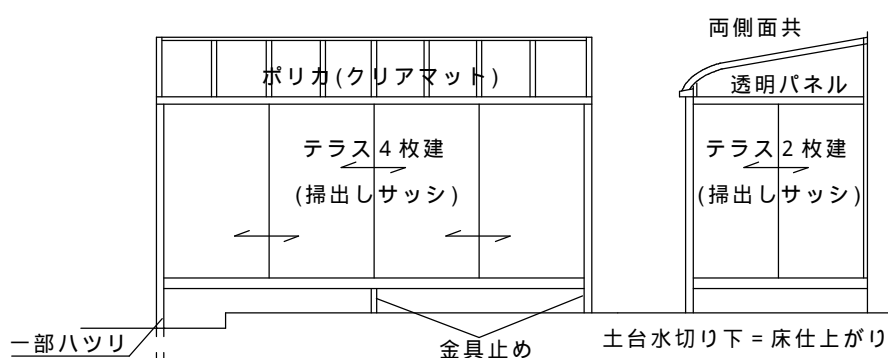
サニージュ立面図
