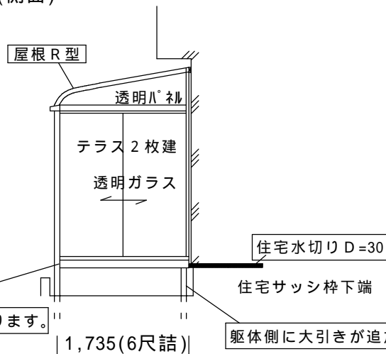
側面図(側面)
