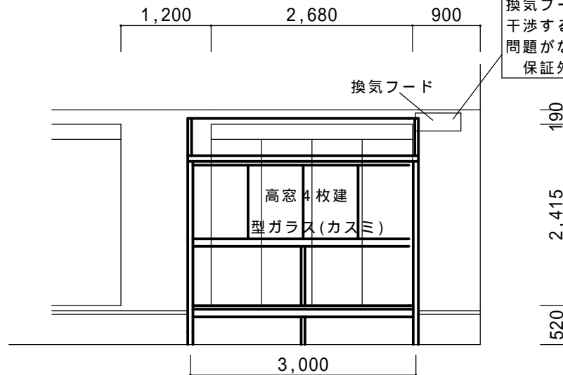
立面図(前面)
