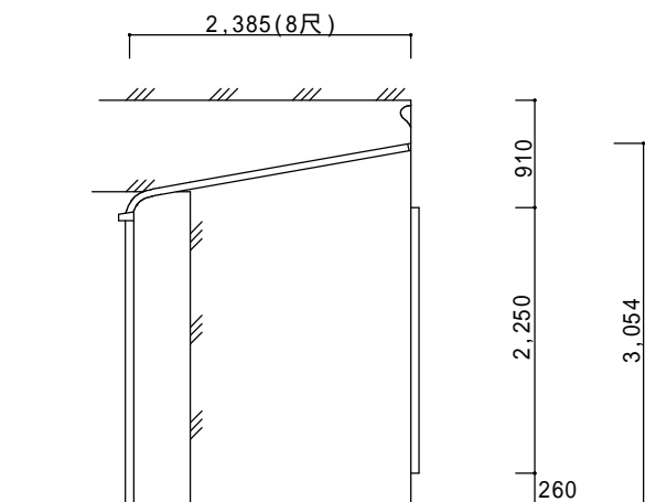
立面図(側面)
