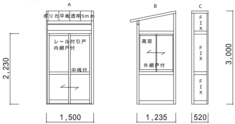
立面図
