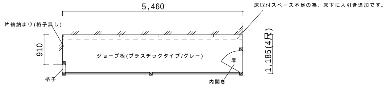
平面図（ビューステージFスタイル、出幅4尺）
