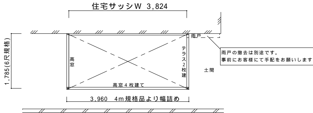
平面図
