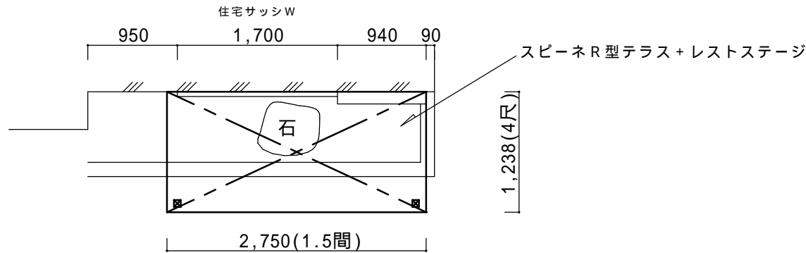
平面図
